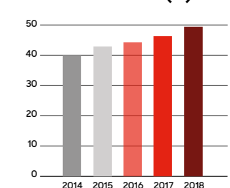
Omavaraisuusaste (%)
