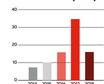
Bruttoinvestoinnit (MEUR)
