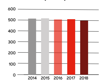
Liikevaihto (MEUR)
