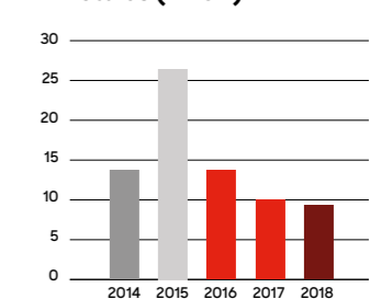
Liiketulos (MEUR)
