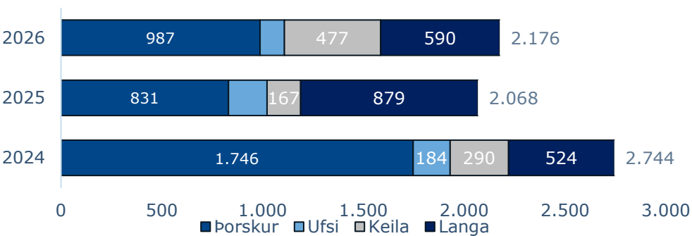
Móttaka saltfiskvinnslna
