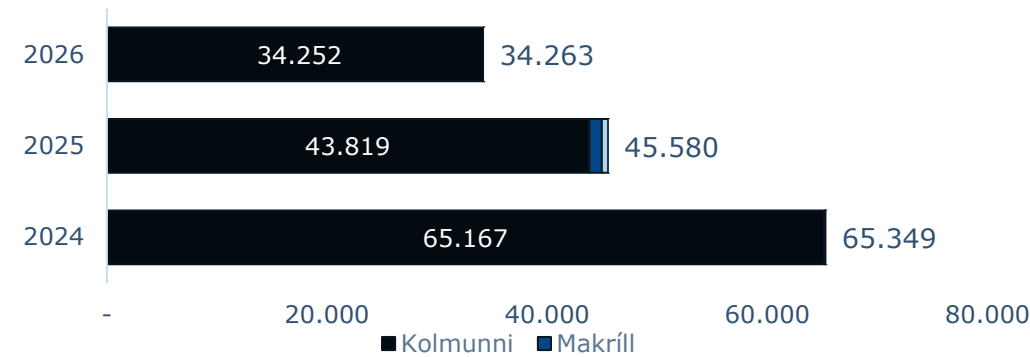
Móttaka fiskimjölsverksmiðja
