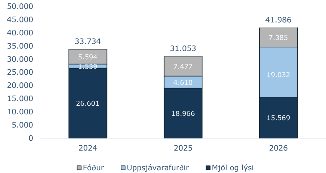
Framleiðsla afurða
