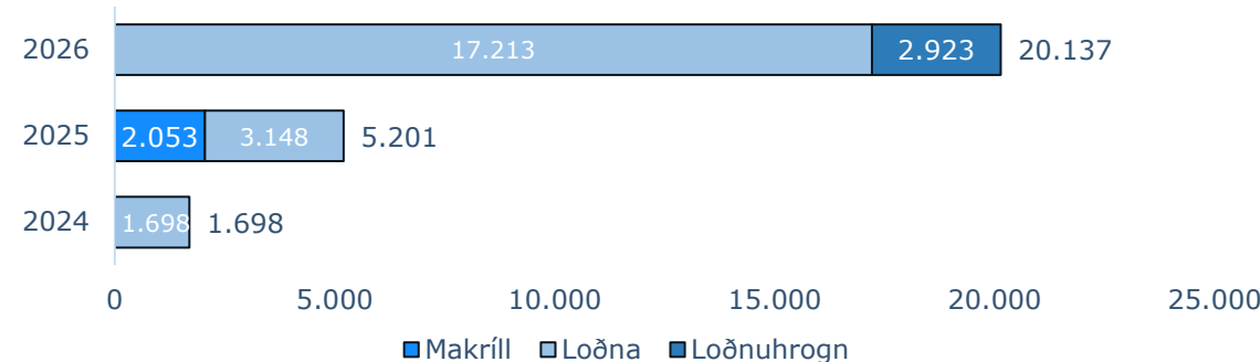
Móttaka uppsjávarfrystingar
