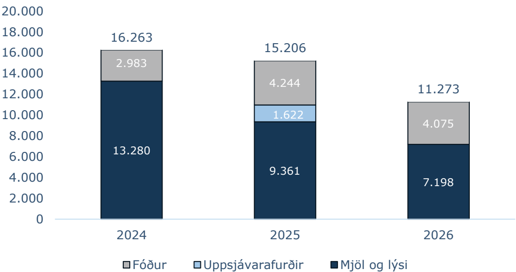
Framleiðsla afurða
