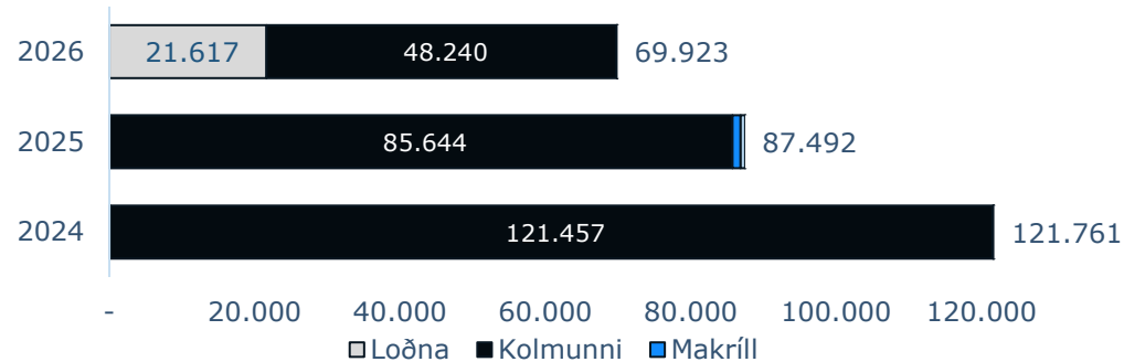
Framleiðsla afurða
